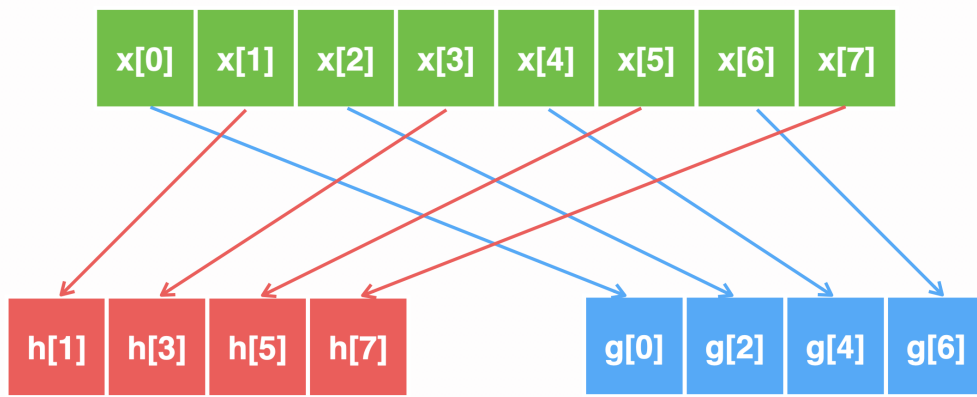
Рис. 2 – Прореживание сигнала по времени
